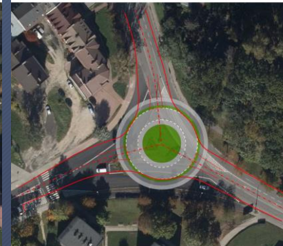
STARACHOWICE - PRZEBIEG DROGI WOJEWÓDZKIEJ NR 744 PRZEZ MIASTO PROPOZYCJE PRZEBUDOWY SKRZYŻOWAN skrzyżowanie al. Armii Krajowej / Iłżecka przebudowa skrzyżowania na rondo (średnica zewn. 30 m) powiększenie ronda z wyspa i regulacja własności
