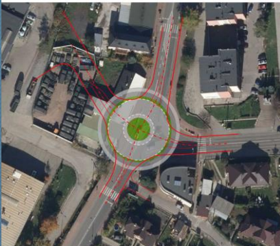
STARACHOWICE - PRZEBIEG DROGI WOJEWÓDZKIEJ NR 744 PRZEZ MIASTO PROPOZYCJE PRZEBUDOWY SKRZYŻOWAN skrzyżowanie al. Armii Krajowej / Wojska Polskiego przebudowa skrzyżowania na rondo (średnica zewn. 30 m)
