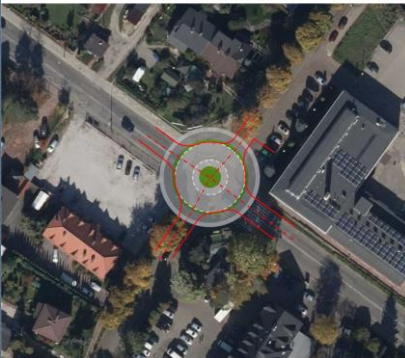
STARACHOWICE - PRZEBIEG DROGI WOJEWÓDZKIEJ NR 744 PRZEZ MIASTO PROPOZYCJE PRZEBUDOWY SKRZYŻOWAN Rondo "Solidarności" regulacja pasa drogowego i własności terenu
