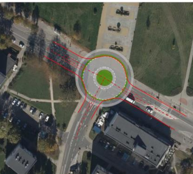
STARACHOWICE - PRZEBIEG DROGI WOJEWÓDZKIEJ NR 744 PRZEZ MIASTO PROPOZYCJE PRZEBUDOWY SKRZYŻOWAN skrzyżowanie al. Armii Krajowej / Wojska Polskiego przebudowa skrzyżowania na rondo (średnica zewn. 30 m)
